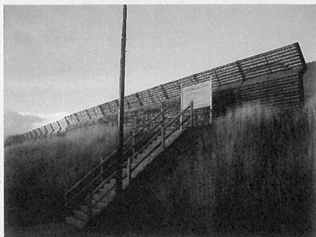
北海道野付郡別海町中春別「カラマツ間伐材による防雪柵」
